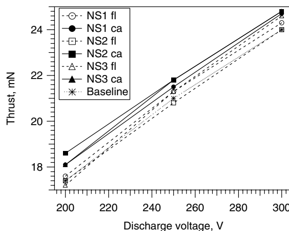
Fig. 11 Thrust ( \pm 1 mN) for configurations NS1, NS2, NS3, and the baseline.
